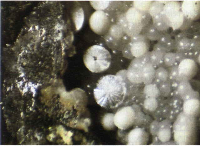
Abb. 3a: Kugelige Koninckit-Aggregate, radialstrahlig aufgebaut, im Quer- schnitt bis 0,3 mm. Fundort: Gunders- dorfer Almstraße bei Oberbuchach im Gailtal (Karnische Alpen). Foto u. Sammlung: M. Puttner.
